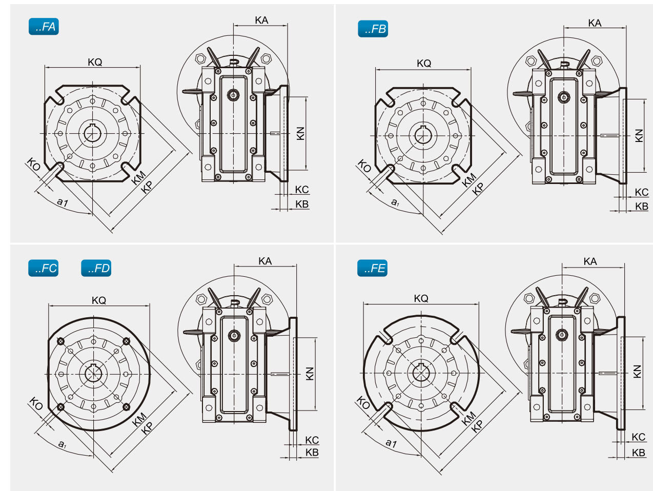
OTS..F 输出法兰尺寸/Output Flange Dimension
