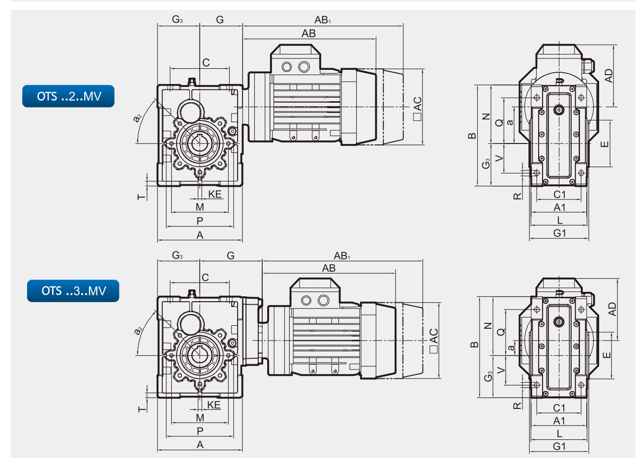
OTS ..MV.. 外形尺寸 / Outline Dimension
