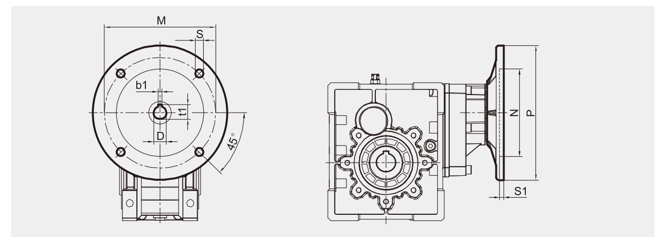
OTS..IEC 输入法兰尺寸/Input Flange Dimension
